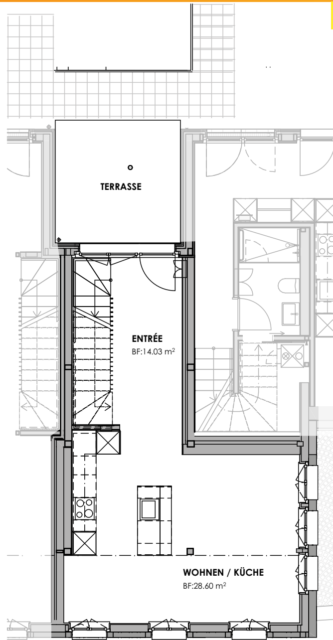
Erdgeschoss
